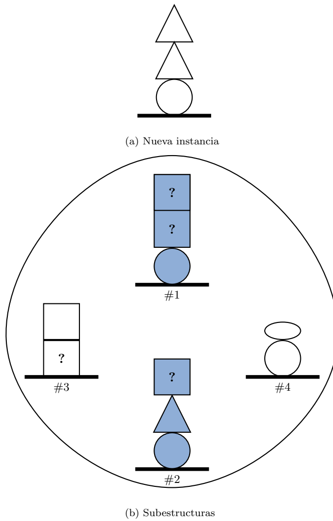
Figura 3.16: Ejemplo de predicción para nuevas instancias. La instancia dada en (a) está cubierta por las subestructuras pintadas en celeste
