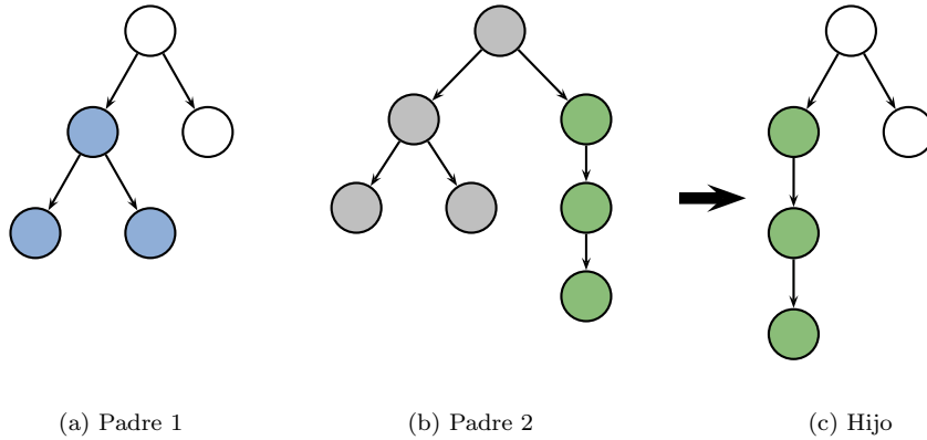
Figura 3.5: Operación de cruce de un algoritmo de PG
