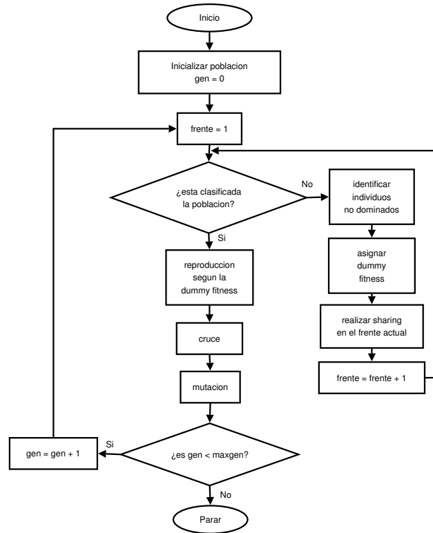
Figura 2.11: Diagrama de flujo del algoritmo NSGA
