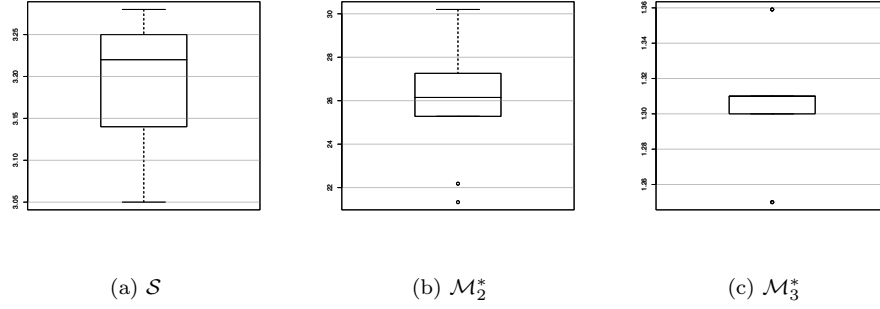
Figura 3.12: Boxplots de las métricas \mathcal{S} , \mathcal{M}_2^* y \mathcal{M}_3^* para el CC-EMO en el dominio geométrico
