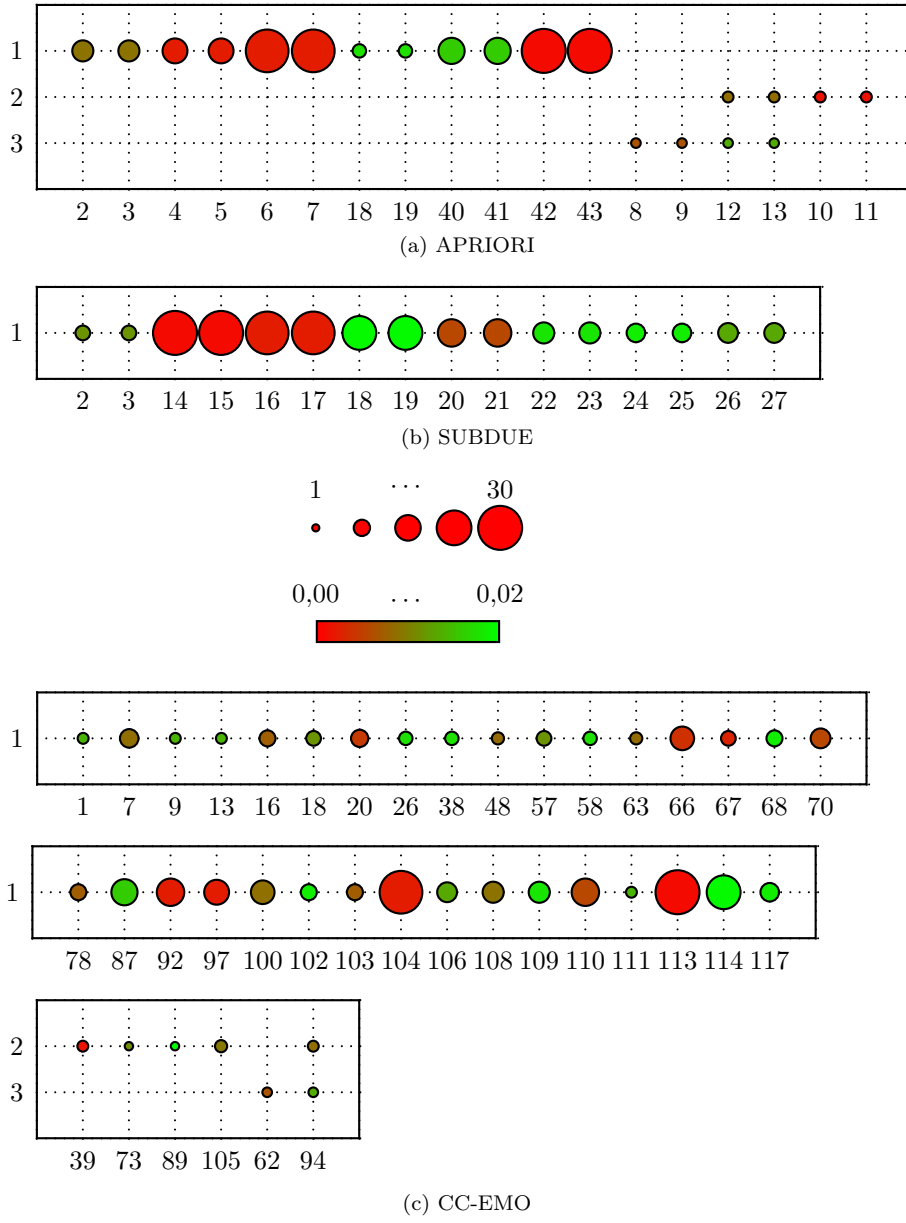
Figura 4.9: Intersección de los ClustersA y ClustersB para APRIORI, SUBDUE y CC-EMO.
