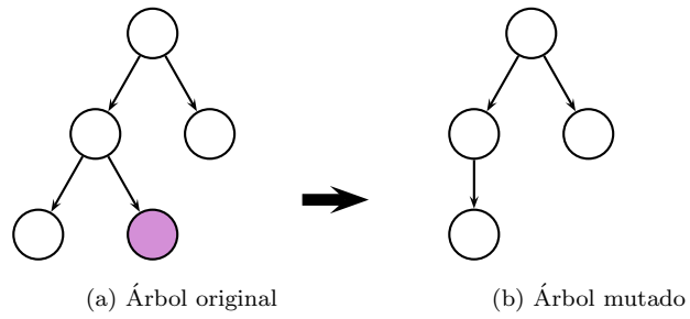
Figura 3.6: Mutación: borrado de una hoja
