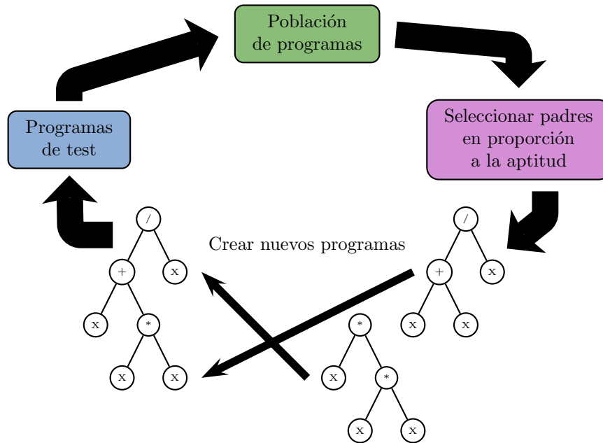
Figura 2.9: Ciclo de PG
