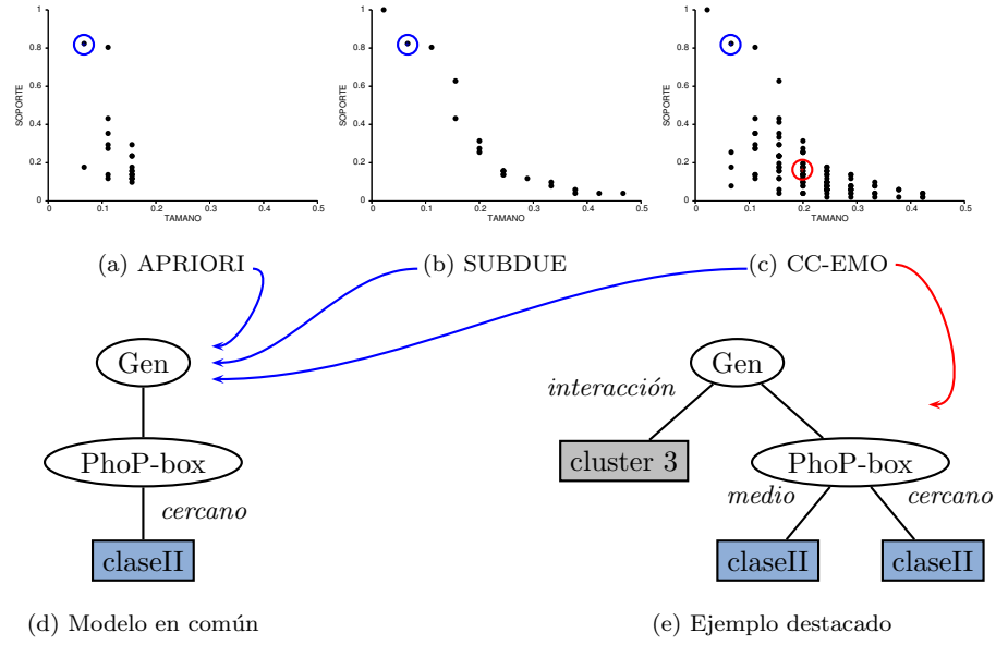
Figura 4.5: Frentes de Pareto para el dominio de regulación genética en procariotas.
