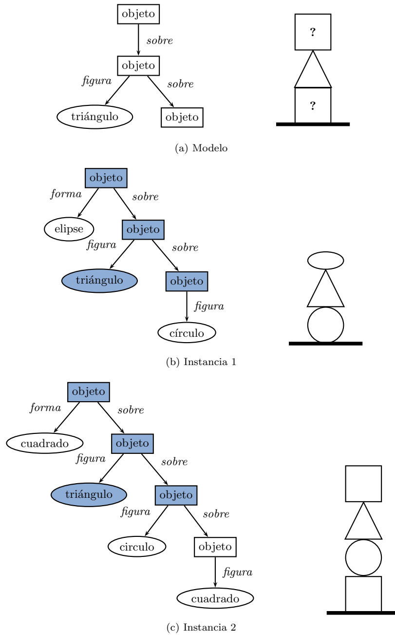
Figura 3.9: Ejemplos de cobertura de una subestructura (a) a dos instancias (b,c)
