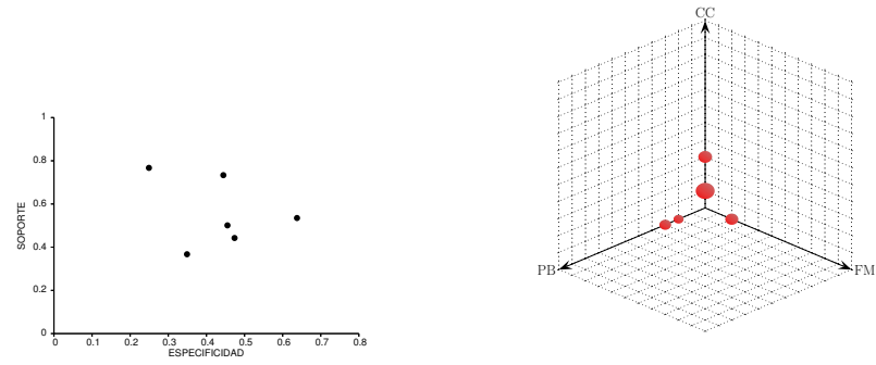
(a) APRIORI
