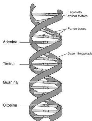
Figura 1.6: Doble hélice
