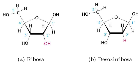
Figura 1.3: Azúcares
