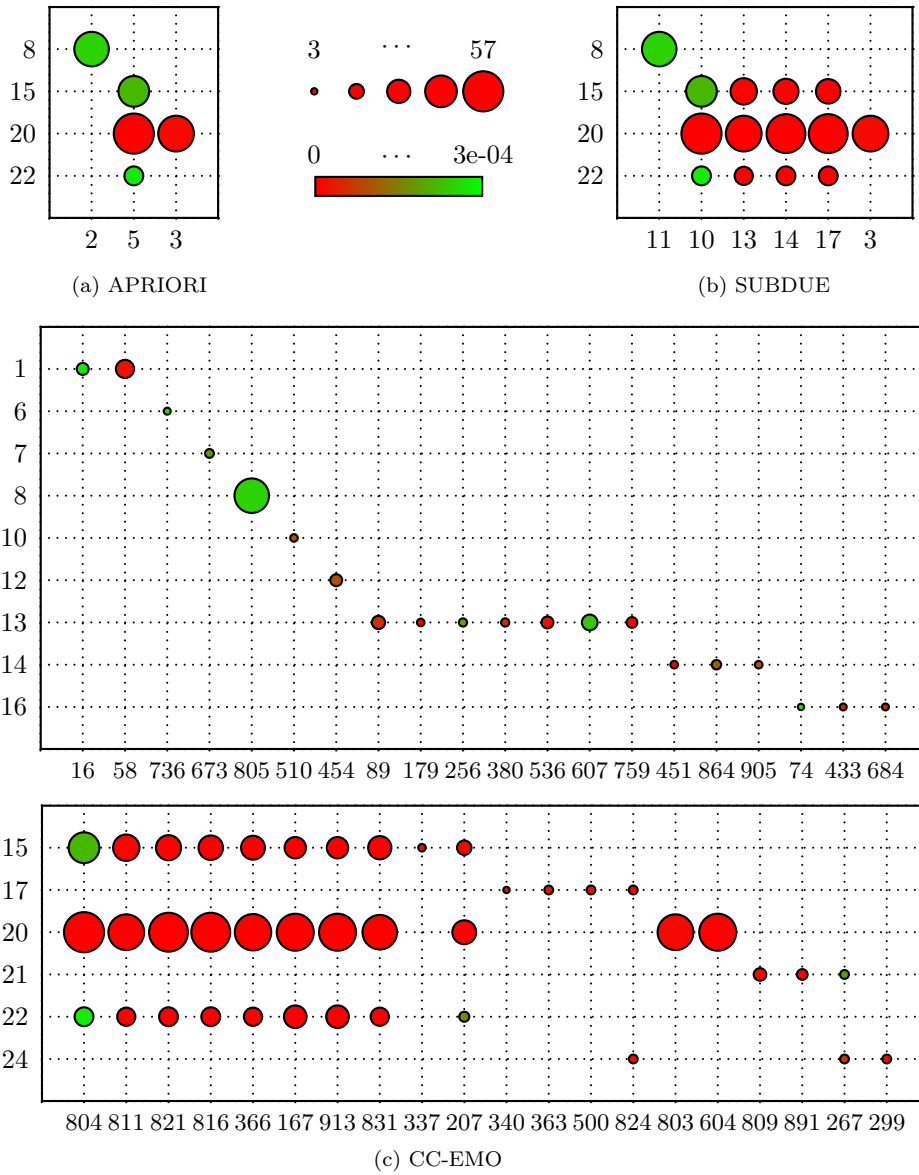
Figura 5.11: Intersección de los ClustersA y ClustersB para APRIORI, SUBDUE y CC-EMO. No se muestran todas las intersecciones de CC-EMO en esta gráfica, el gráfico completo se encuentra en el Apéndice A.1.
