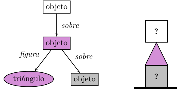
Figura 3.3: Ejemplo de subestructuras del dominio geométrico
