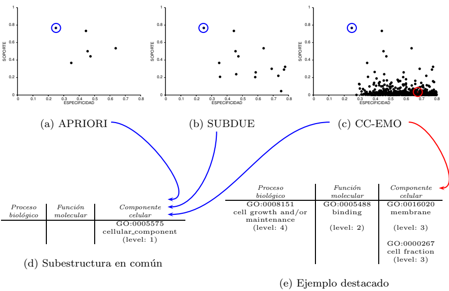
Figura 5.7: Frentes de Pareto para el dominio de ontología de genes .
