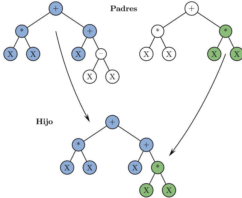
Figura 2.8: x^2 + (x + (x - x)) cruzado con 2x^2 para producir 2x^2 + x
