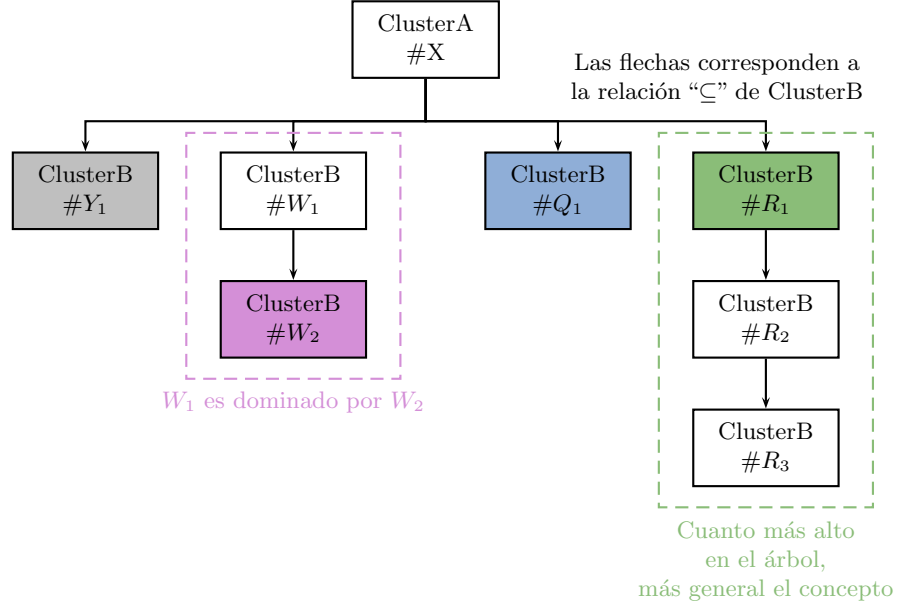
Figura 3.15: Ejemplo de compactación. La jerarquía viene dada por la relación entre los ClusterA y ClusterB. Los clusters coloreados corresponden a aquellos que se mantienen finalmente.
