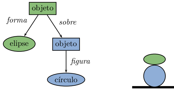
Figura 3.2: Ejemplo de instancia de la base de datos de objetos estructurados del dominio geométrico
