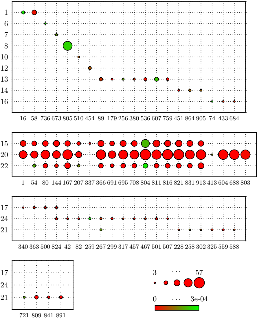
Figura A.1: Intersección de ClustersA y ClustersB para CC-EMO. El gráfico representa cada intersección como un círculo, cuyo tamaño crece con la cantidad de elementos en la intersección entre los clusters, mientras que el color muestra el p-value de la intersección.
