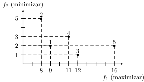
Figura 2.10: Dominancia entre soluciones.
