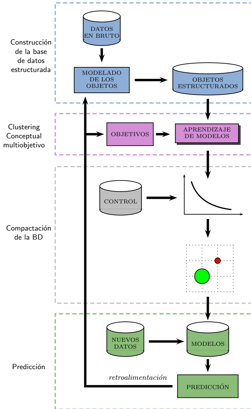
Figura 3.1: Esquema general de la metodología CC-EMO
