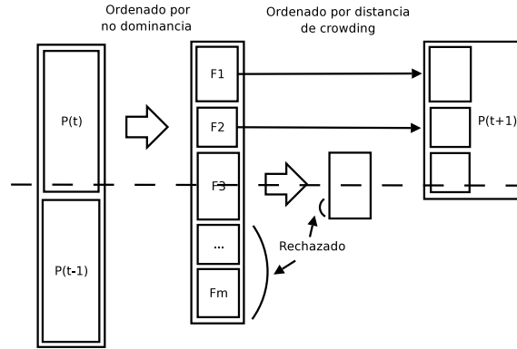
Figura 2.12: Esquema del algoritmo NSGA-II
