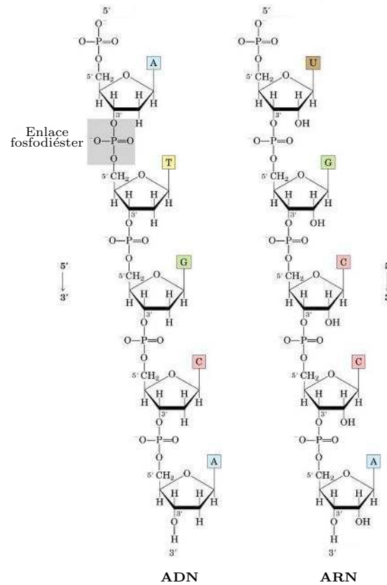
Figura 1.7: Polinucleótidos
