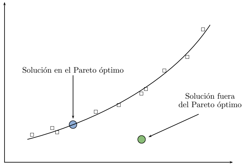
Figura 2.13: Soluciones posibles
