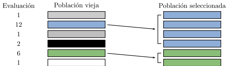
Figura 2.6: Ejemplo de aplicación del mecanismo de selección
