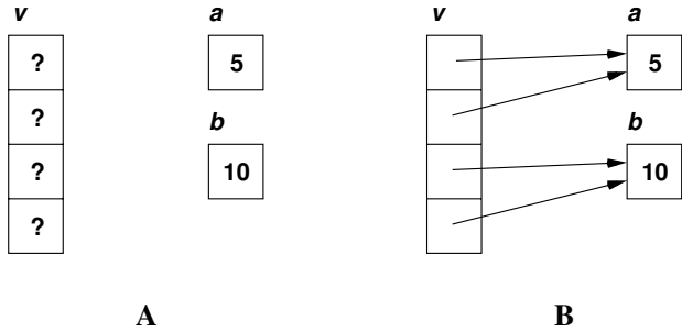
Estado de la memoria: A) tras la declaración, B) tras la iniciación de los v[i].
