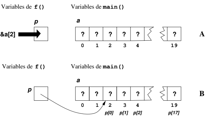
A) Correspondencia entre parámetros actuales y formales el la llamada a f(). B) Estado de la memoria tras establecer la correspondencia entre parámetros actuales y formales.
