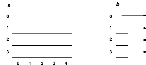
Representación en memoria de la matriz int a[4][5] y del vector int *b[4]
