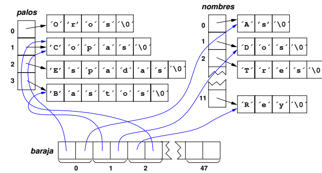
Estado de la memoria para una ordenación particular de cartas
